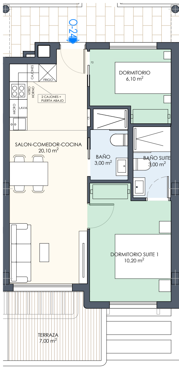
PLANTA PRIMERA
